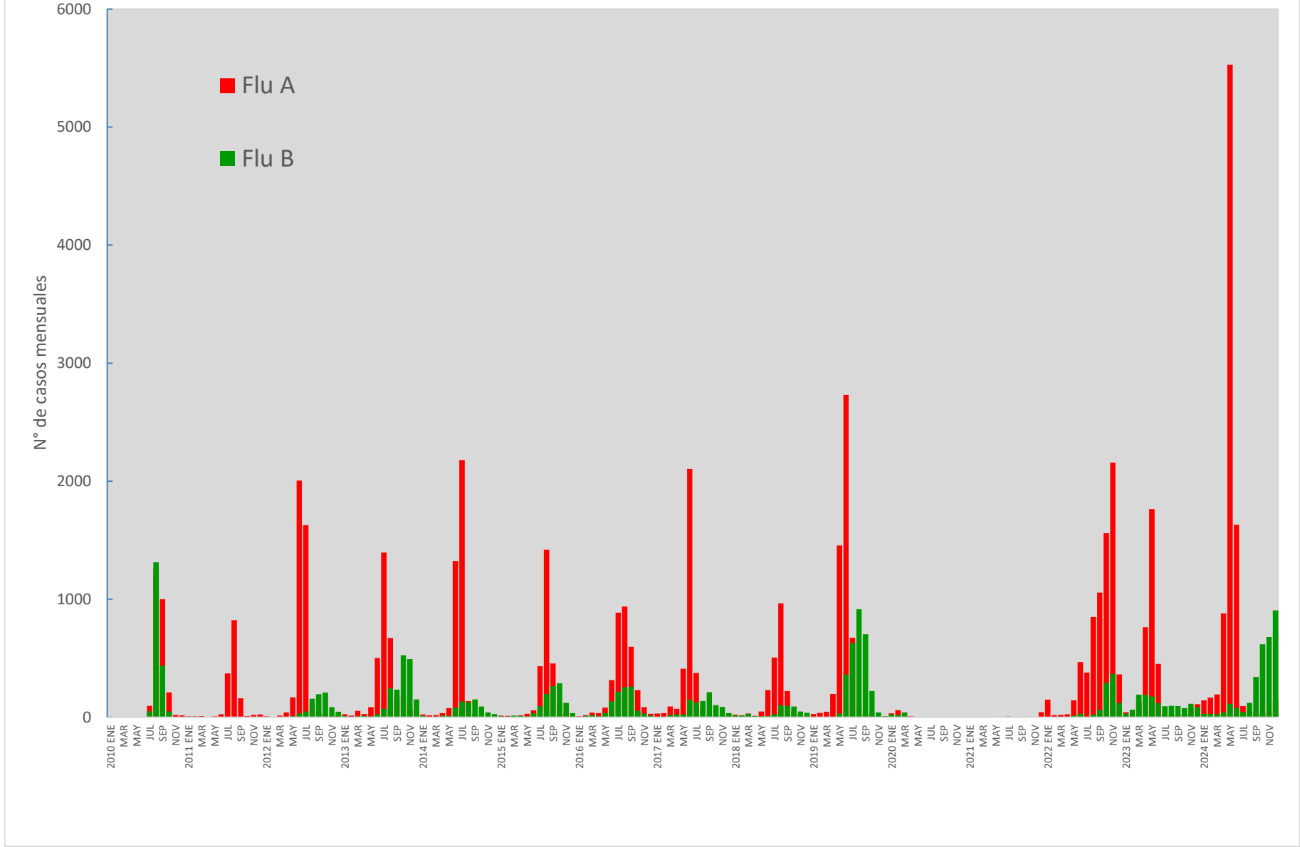
Circulación de influenza A y B, Región Metropolitana. 2010-2024
